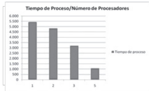
Figura 14. Tiempo de proceso consumido por el cluster usando 10000 pares de bases comparado con los procesadores en los cuales se hizo el corrimiento
