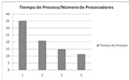
Figura 13. Tiempo de proceso consumido por el cluster usando 1000 pares de bases comparado con los procesadores en los cuales se hizo el corrimiento
