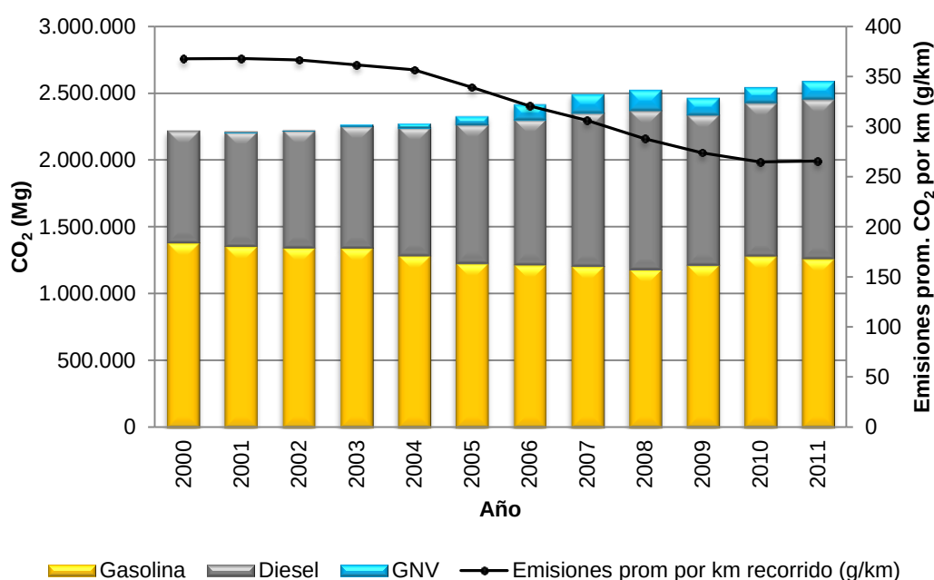
Figura 4.10. Evolución de las emisiones de dióxido de carbono (CO 2 )
