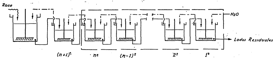
DIAGRAMA ESQUEMATICO DE UNA BATERIA DE EXTRACTORES
