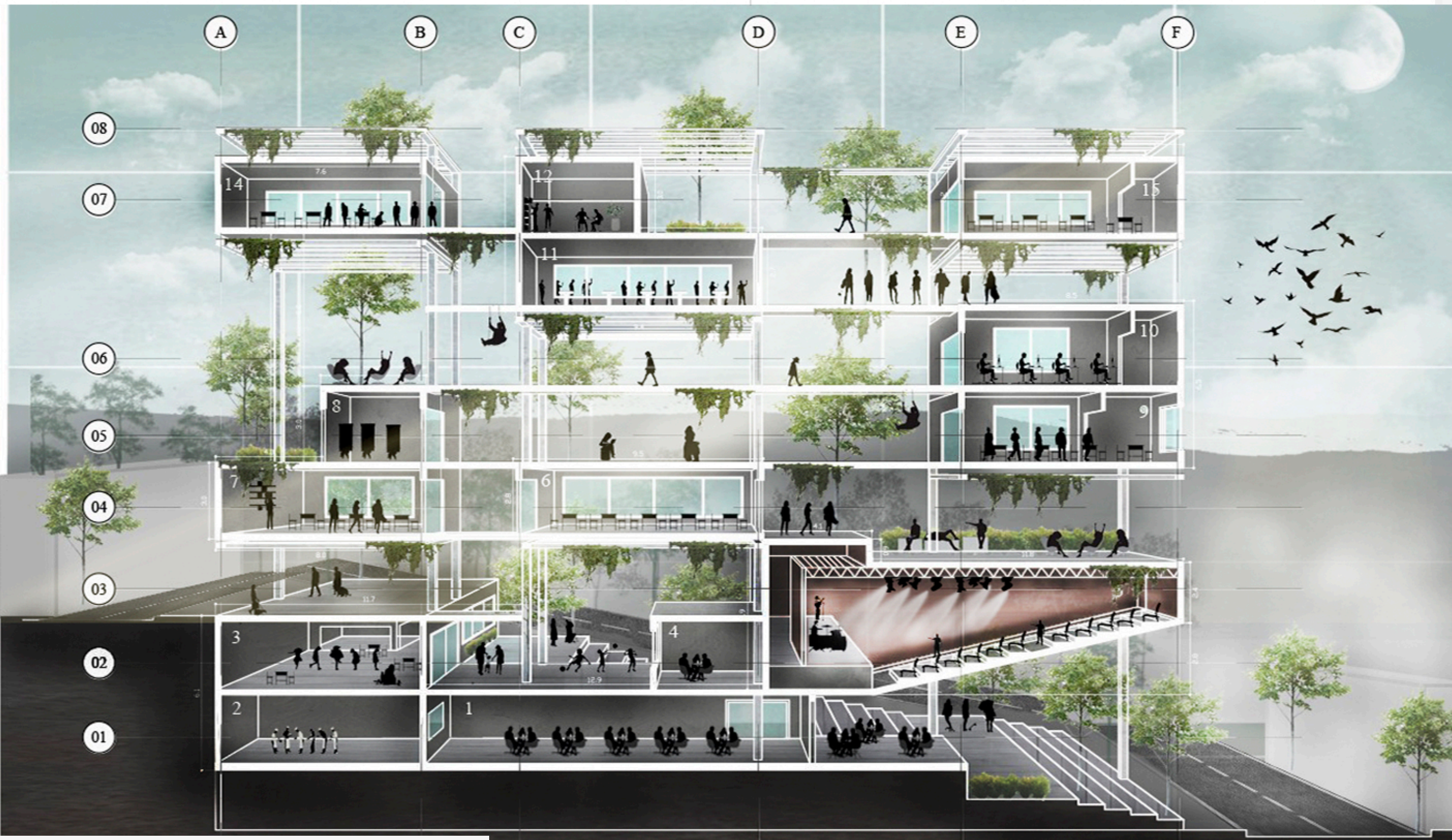
SECCION PRINCIPAL (ESCALA 1:125)
