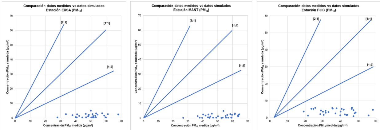
Figura 6. Comparación datos medidos estación de monitoreo vs datos simulados con CAMx para el contaminante PM 10 en las estaciones EXSA, MANT y PJIC.
