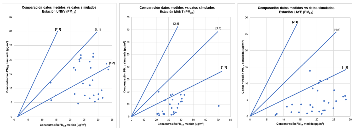
Figura 5. Comparación datos medidos estación de monitoreo vs datos simulados con CAMx para el contaminante PM_{2.5} en las estaciones UNNV, MANT y LAYE.
