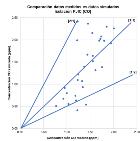
Figura 4. Comparación datos medidos estación de monitoreo vs datos simulados con CAMx para el contaminante CO en la estación PCJIC.
