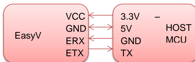
Figura 38. Conexión entre el EasyVR y un Host
