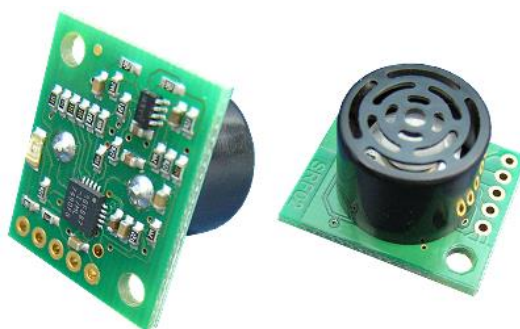
Figura 10. Sensor ultrasónico SRF02, imagen tomada de http://www.robot-electronics.co.uk/htm/srf02tech.htm
