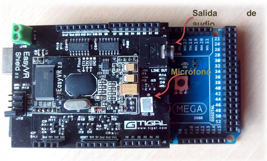
Figura 39. Conexión del Shield EasyVR y Arduino Mega.
