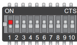
Figura 32. Configuración del DIP Switch en modo RC, imagen tomada de: Datasheet driver RoboClaw 2X30A.
