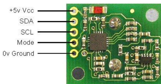
Figura 31. Conexión del sensor SRF02 en modo I2C, imagen tomada de http://www.robot-electronics.co.uk/html/srf02techI2C.htm
