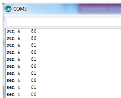
Figura 21. Datos medidos con el objeto ubicado a 80 cm del sensor, imagen tomada de Arduino.
